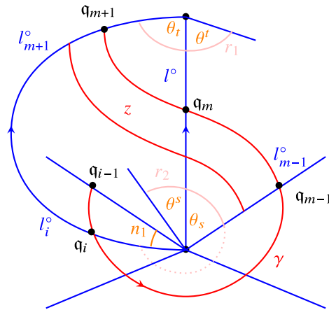
Figure 24. The case |q(l^circ)| = 1 , |q(l_t^circ)| = 1 .
