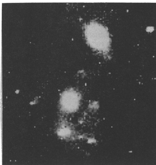
Fig.3c Arp143 (K-Band)
